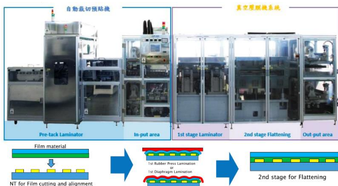
圖 1. 真空壓膜機製程流程
