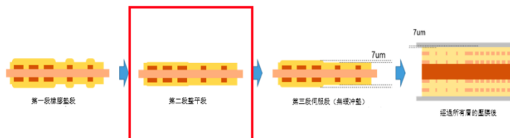
圖 3. 分段壓膜提升製程良率
